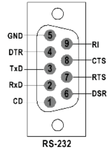
RS-232
