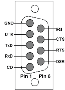
RS-232
