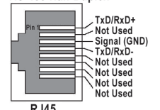
RJ45
