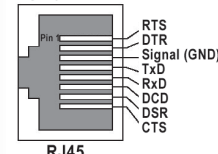
RJ45
