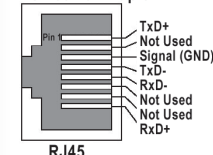
RJ45
